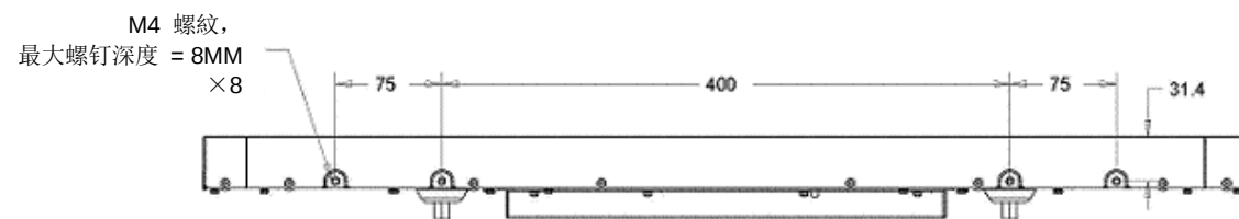
侧面安装水平（顶部/底部）
