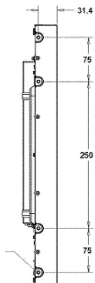
ВЕРТИКАЛЬНЫЙ БОКОВОЙ МОНТАЖ (СЛЕВА/СПРАВА)
